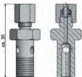
VA Schneidring VA cutting ring
